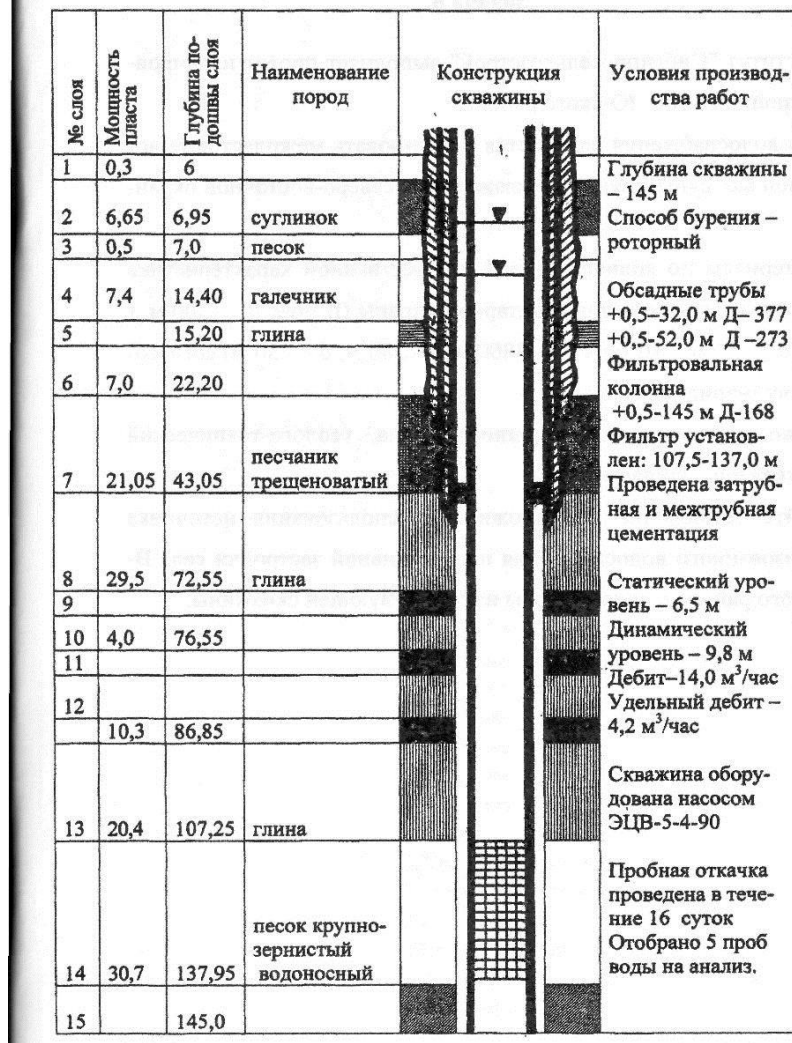
Геолого-технический разрез скважины С-492
